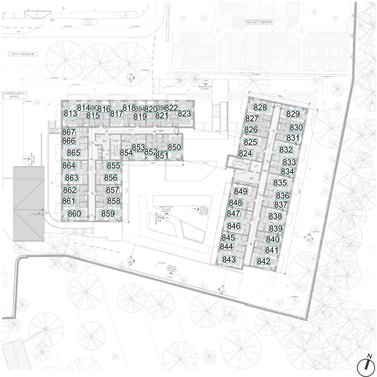
Fig. 33: Floor Plan
