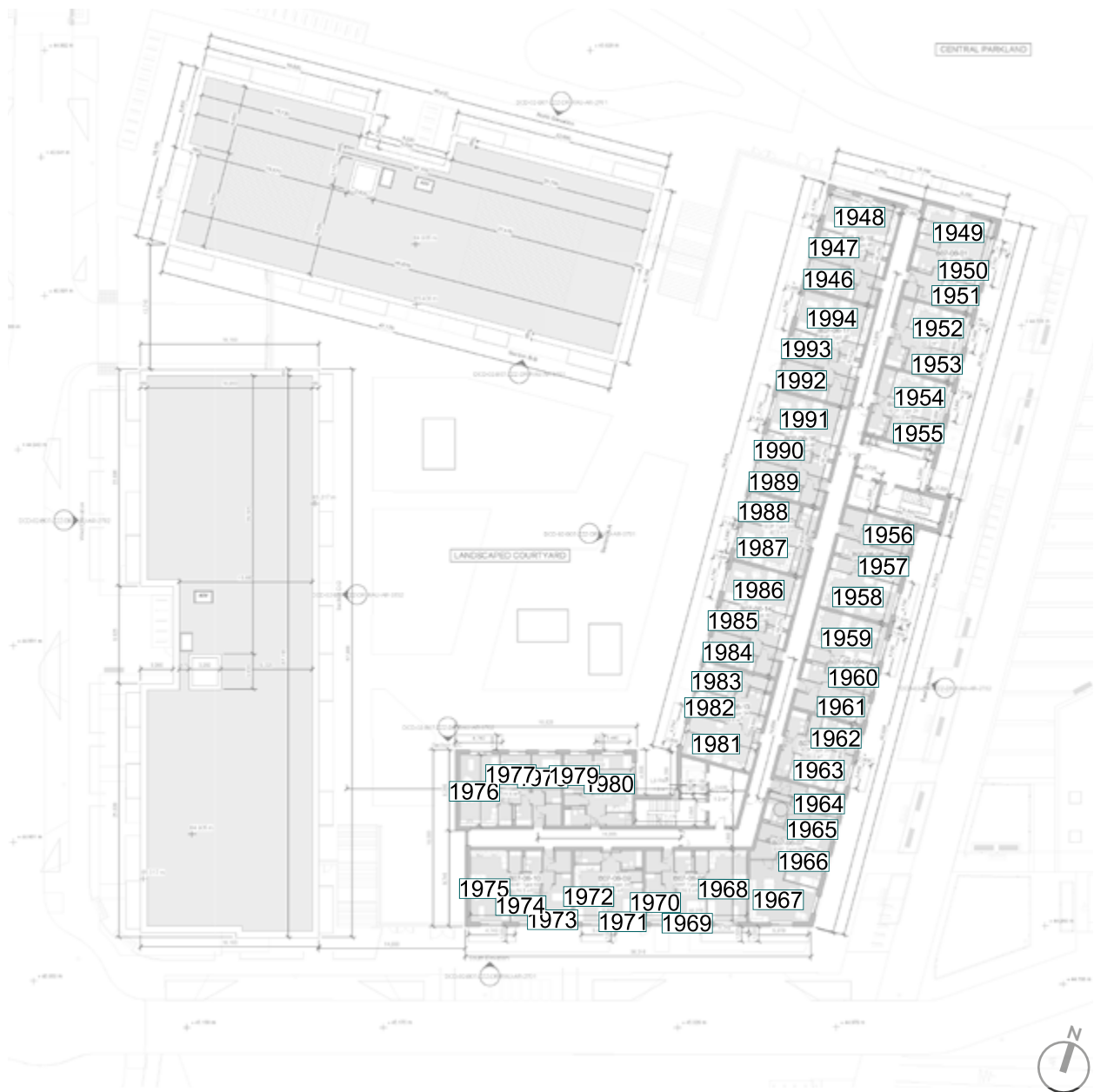
Fig. 64: Floor Plan
